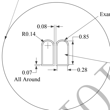
Non Solder Mask Defined Pad
