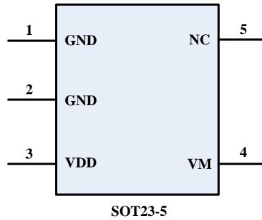
图 2 IP3001 引脚图
