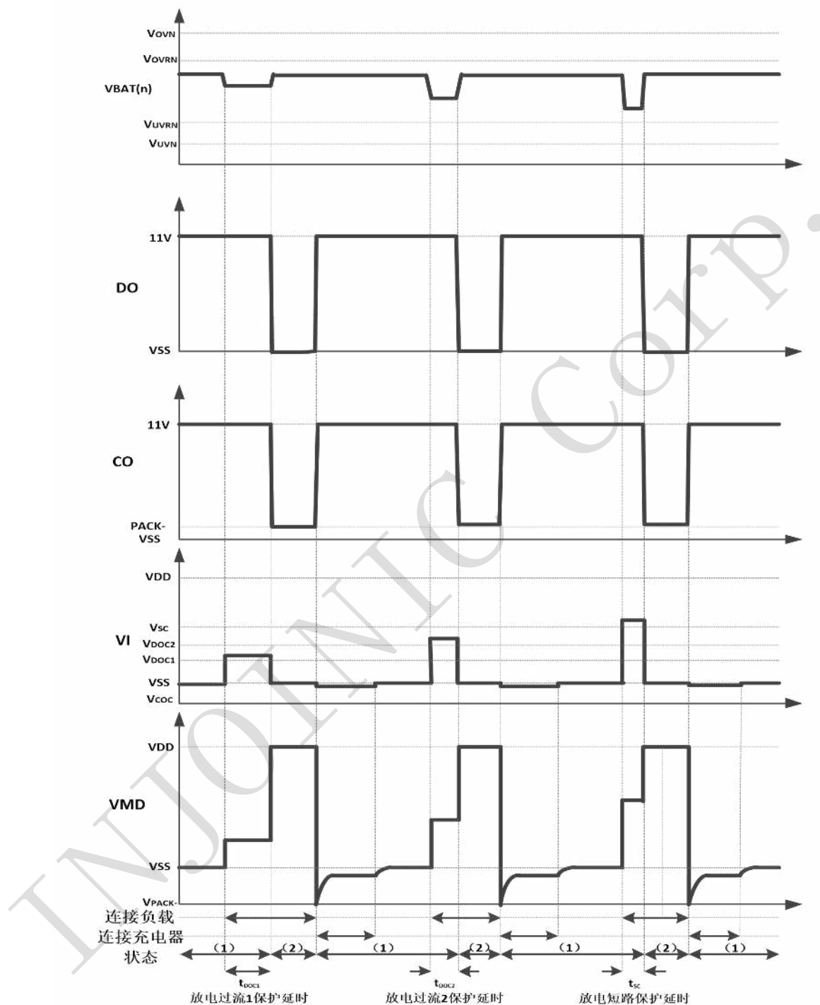
图 5: 放电过流保护解除工作时序图
