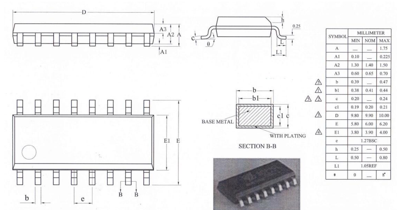
图 14: IP3264 SOP16 封装外形尺寸图
