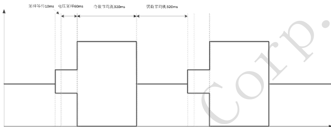
图 4：均衡时序图
