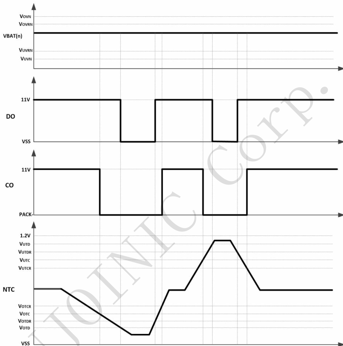
图 9: NTC 高低温保护工作时序图
