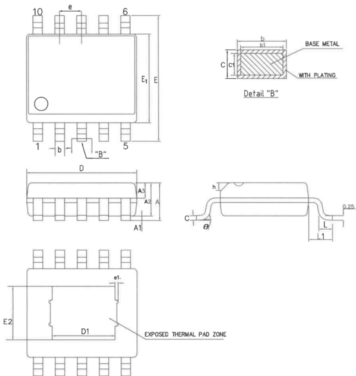
图 11 芯片封装
