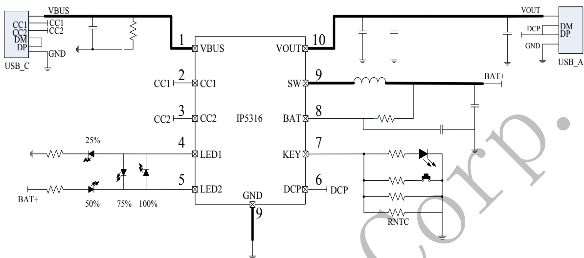
图 1 简化应用原理图(4 LED 指示电量)
