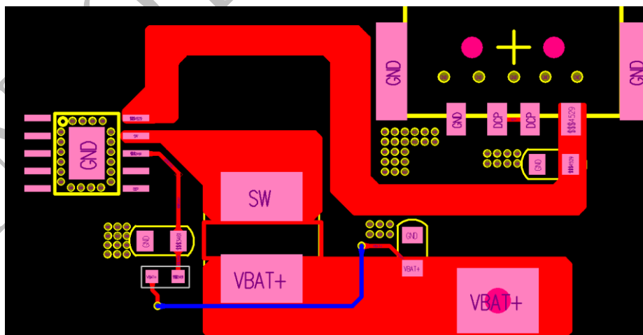
图 9 BAT 电容
