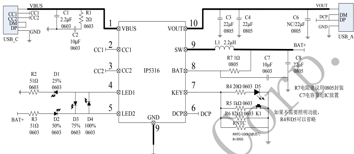
图 10 4LED 电量显示典型应用原理图
