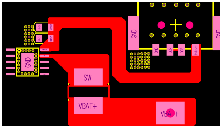
图 8 VOUT 电容
