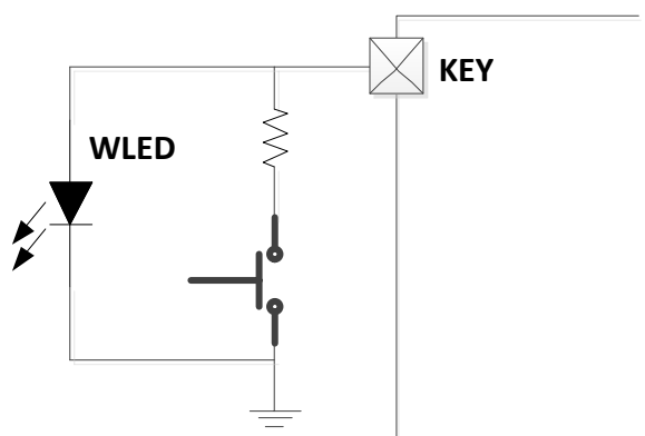
图 3 KEY 按键接法
