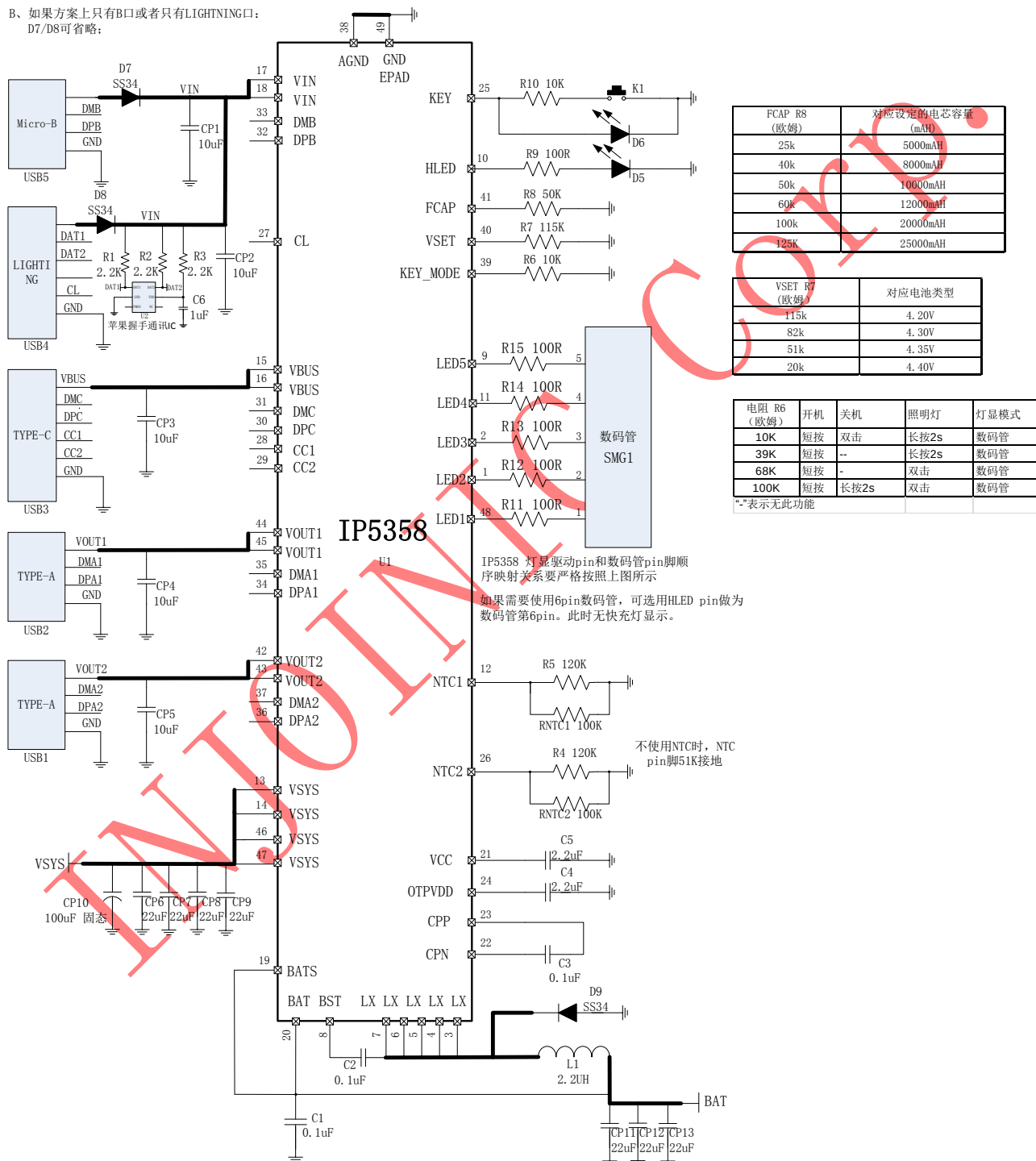
图 17 IP5358 数码管应用的典型应用原理图
