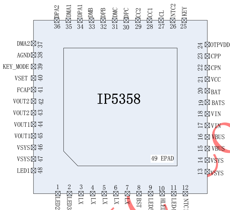
图 2 IP5358 引脚图
