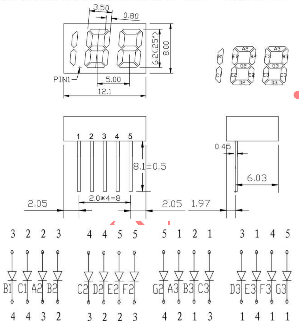
图 13 5pin 188 型数码管电路图
