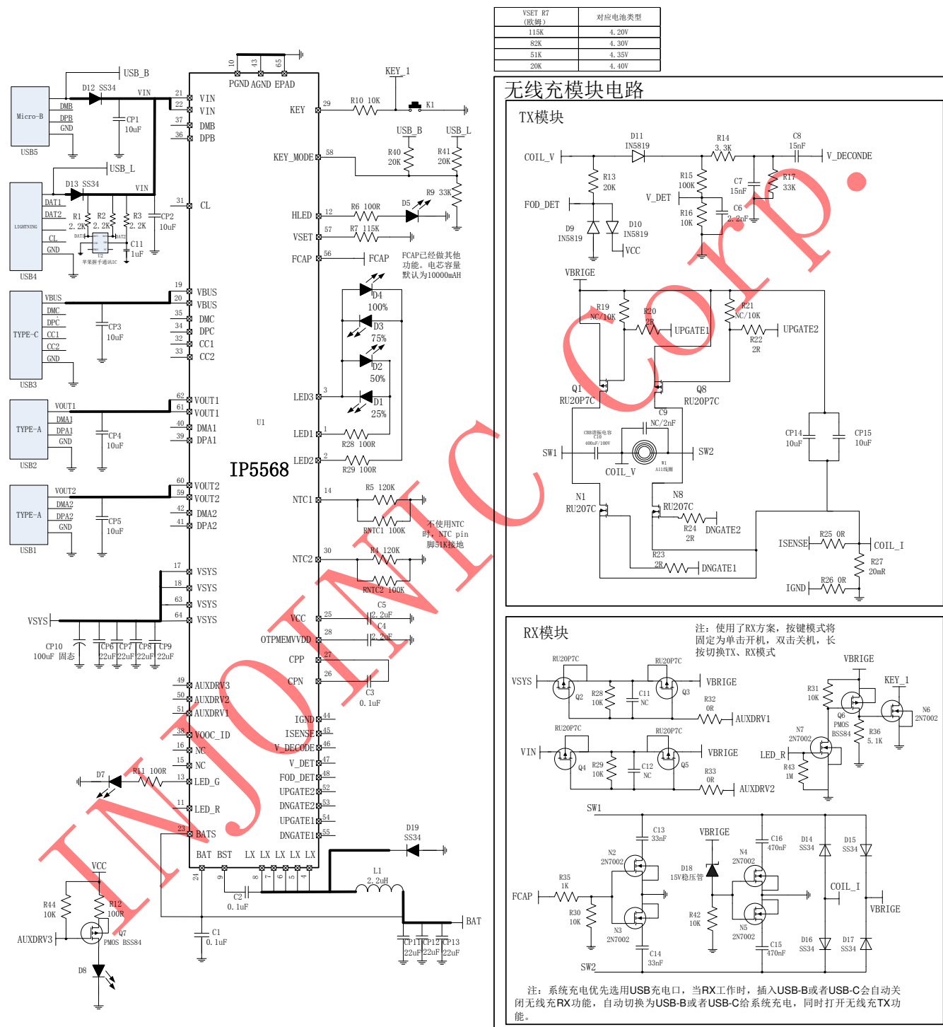
图 18 IP5568_RX_LED 灯应用的典型应用原理图（移动电源+无线充 TX/RX）
