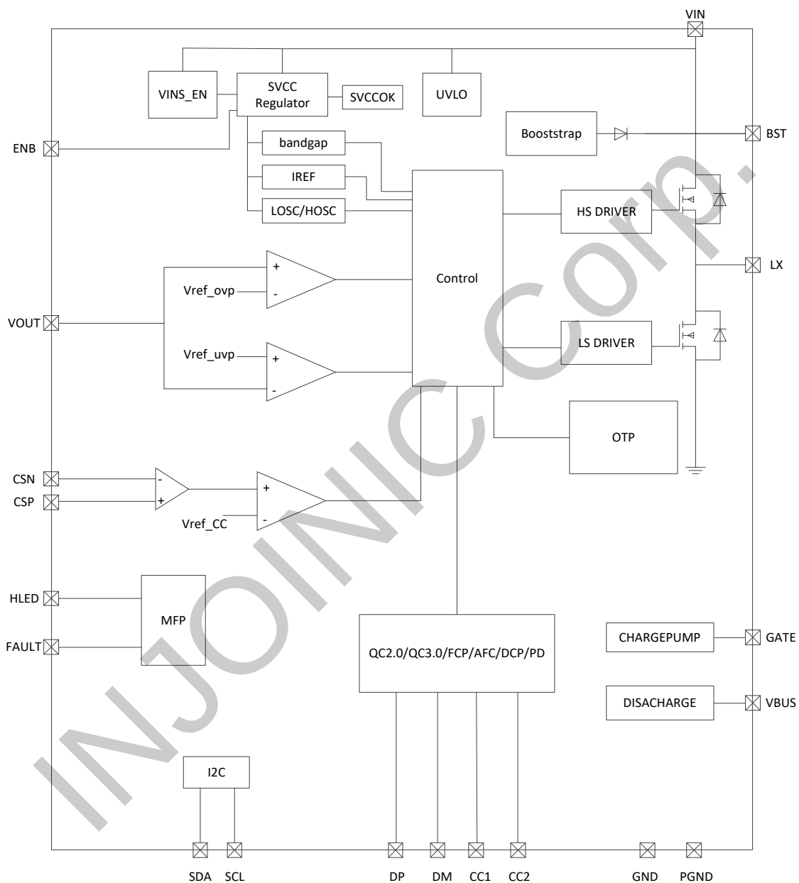
图 4 IP6529 内部框图
