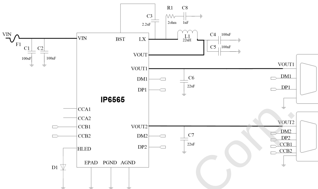
图 2 IP6565_AC USB A 和 USB Type-C 双口快充输出应用原理图
