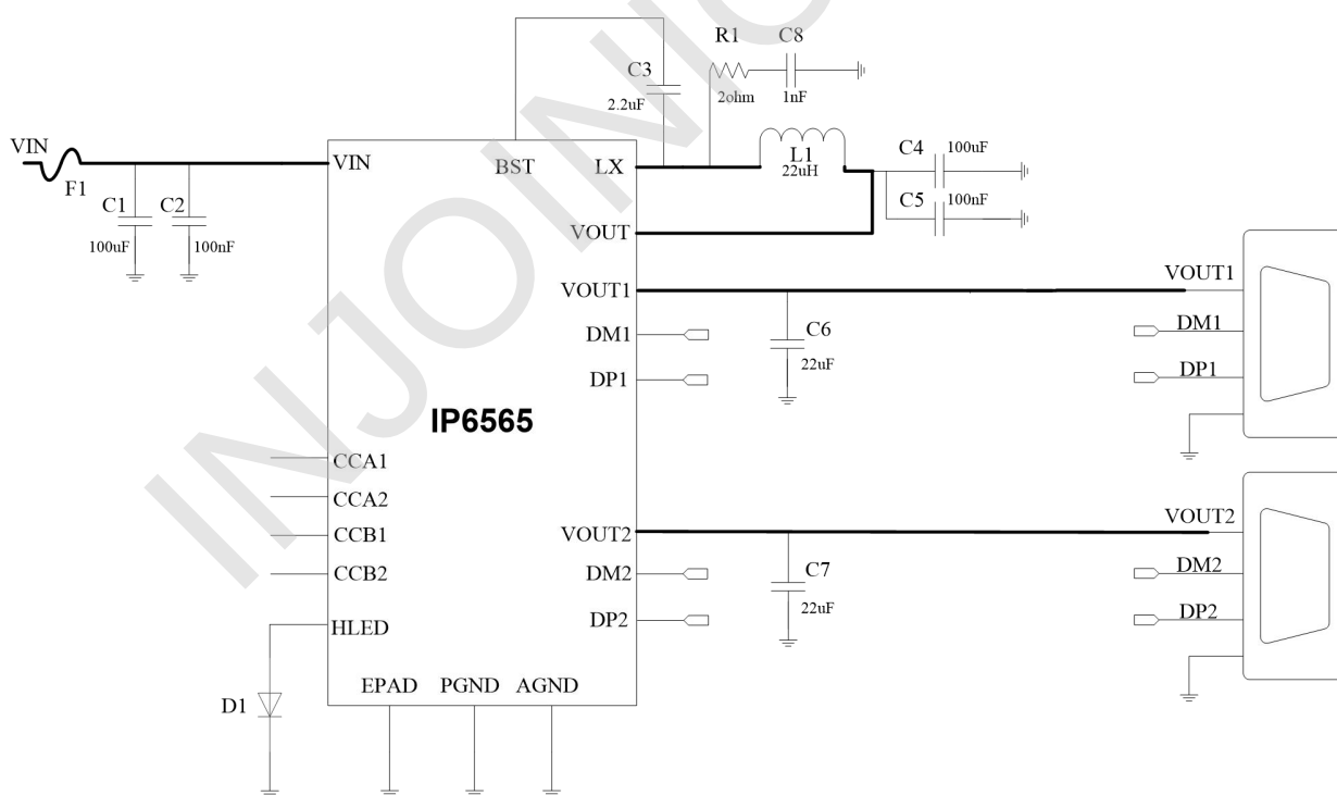
图 3 IP6565_AA 双 USB A 口快充输出应用原理图
