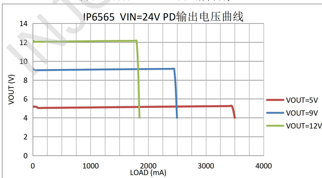
图 7 IP6565 VIN=24V PD 快充 Vout-Iout 输出负载特性曲线
