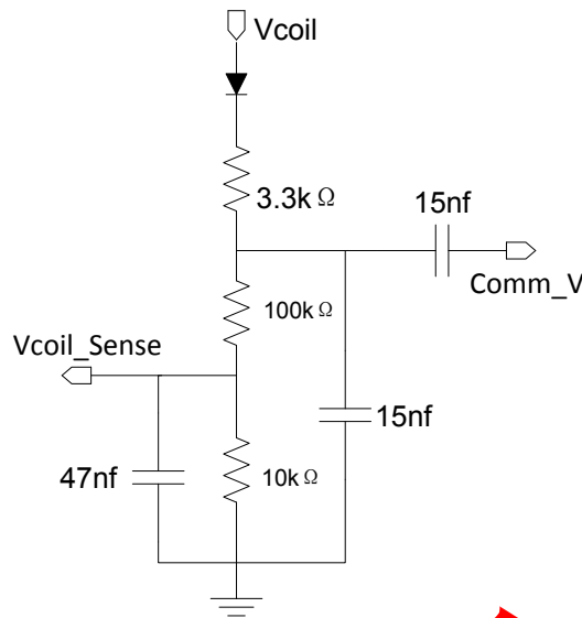
图 4 电压 ASK 解调外围电路
